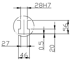
X局部放大視圖 X Section Partview
