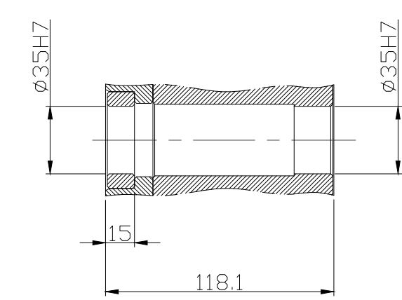
Z-Z剖視圖
