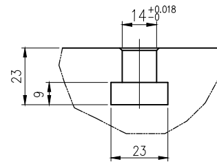
圓盤T槽詳細 (3/1)
